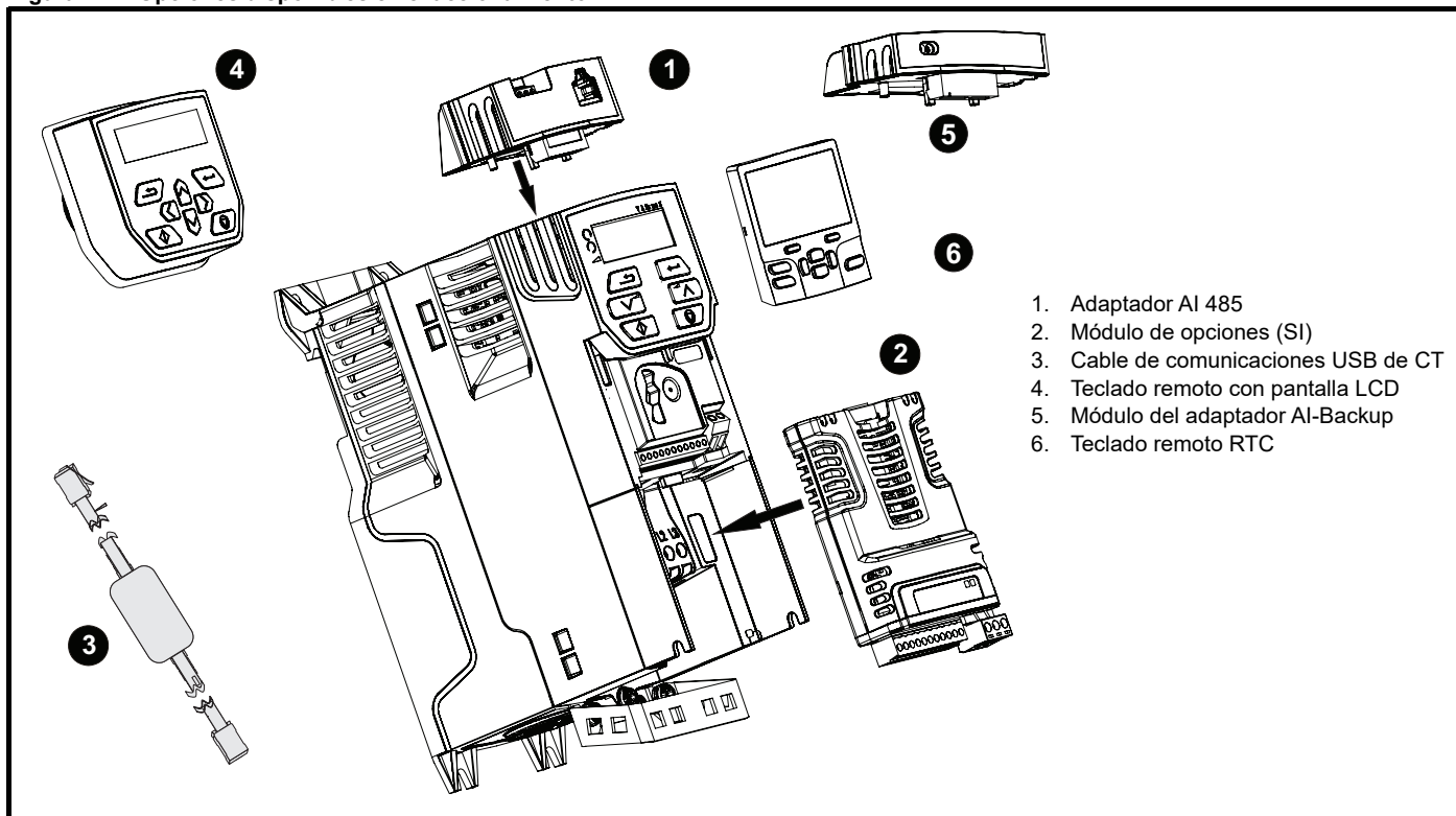
Figura 2-4 Opciones disponibles en el accionamiento
