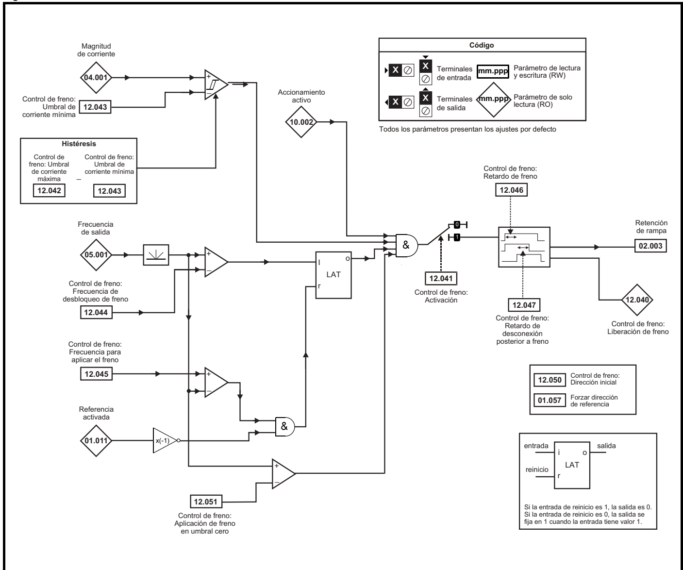
Figura 11-23 Función de freno en bucle abierto
